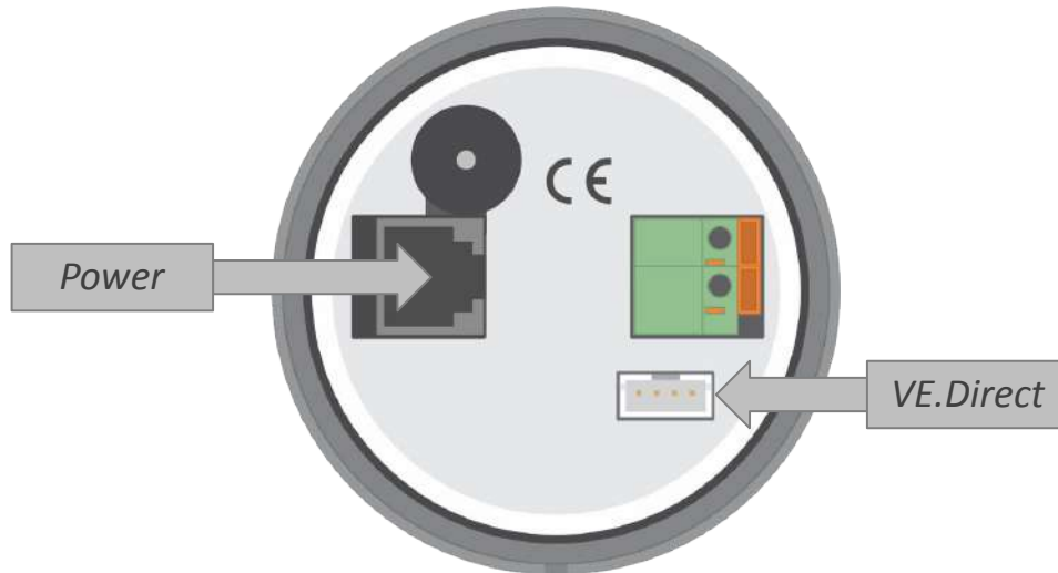
Arrière de l'écran MPPT Control montrant la prise d'alimentation et la connexion VE.Direct
