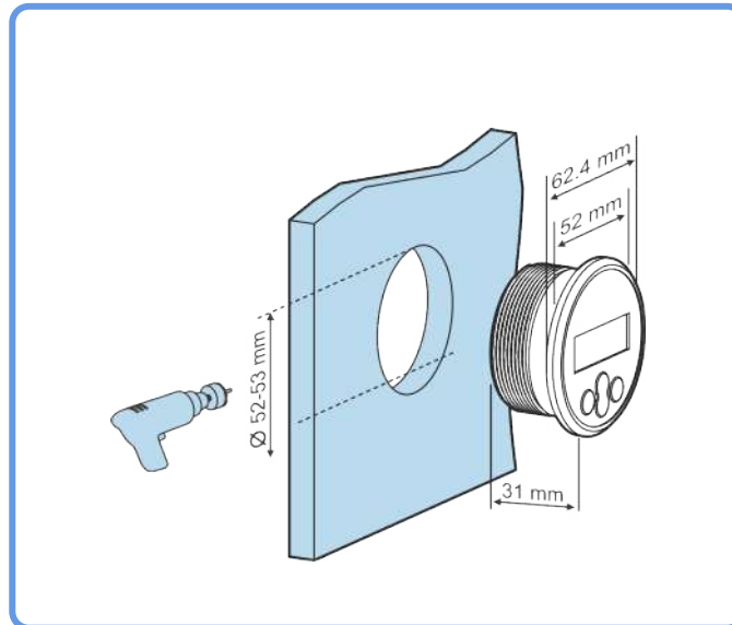
Exigences de largeur et profondeur pour un montage encastré.
