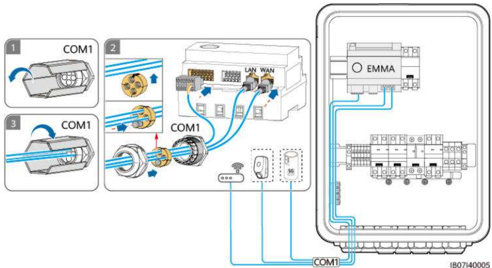
Figure 5-19 Connexion du câble de signal EMMA
