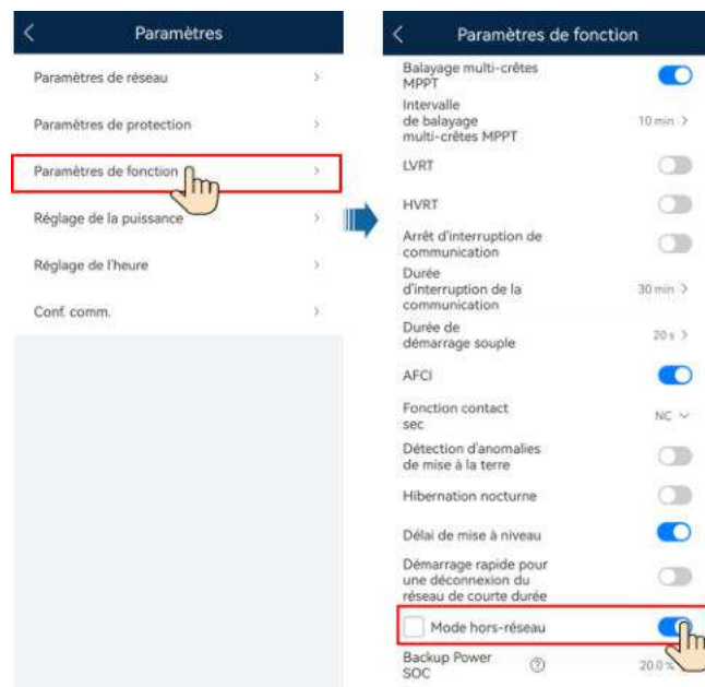
Figure 6-6 Réglage du mode hors-réseau
