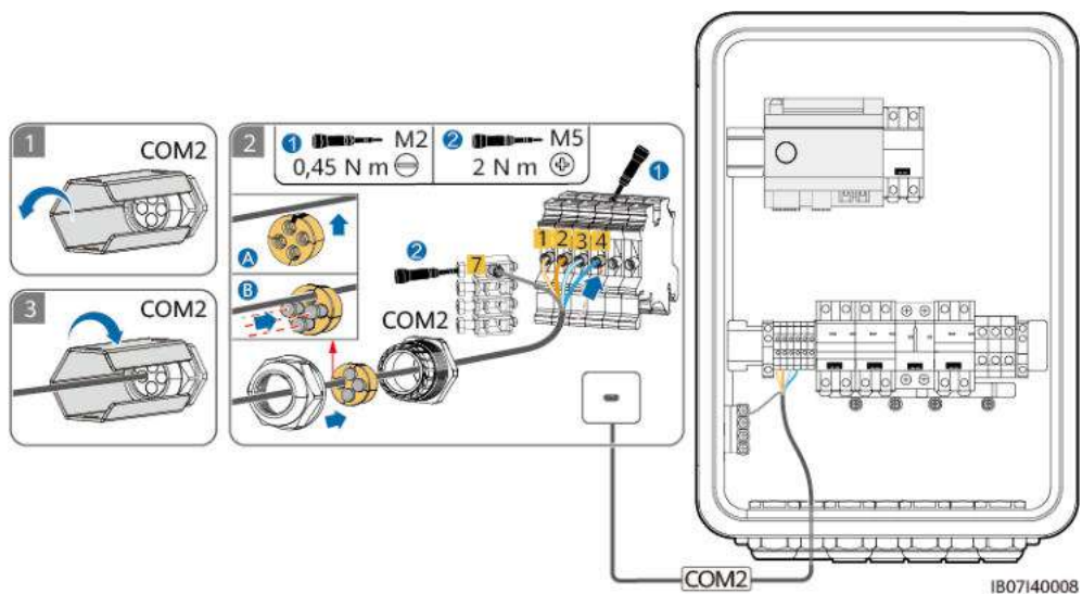
Figure 5-22 Connexion du câble de signal du SmartGuard
