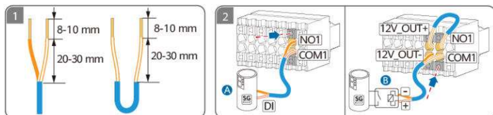
Figure 5-17 Connexion du câble de signal de contrôle de la pompe à chaleur
