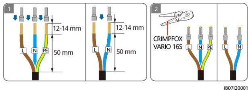
Figure 5-13 Sertissage des bornes d'extrémité du cordon CA
