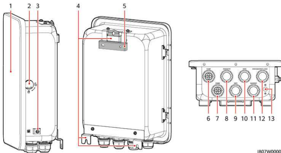
Figure 2-7 Aspect visuel et ports
