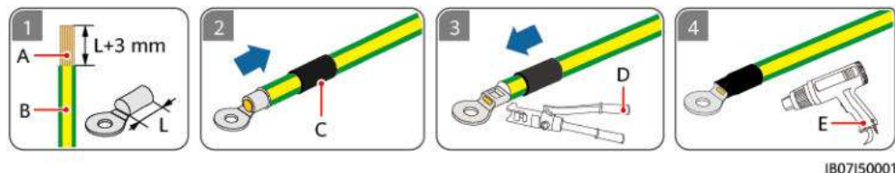
Figure 5-2 Sertissage d'une borne OT
