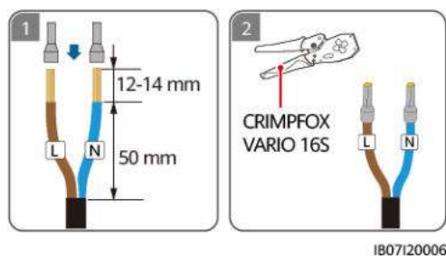
Figure 5-11 Sertissage des bornes d'extrémité du cordon CA SmartGuard-63A-AUS0
