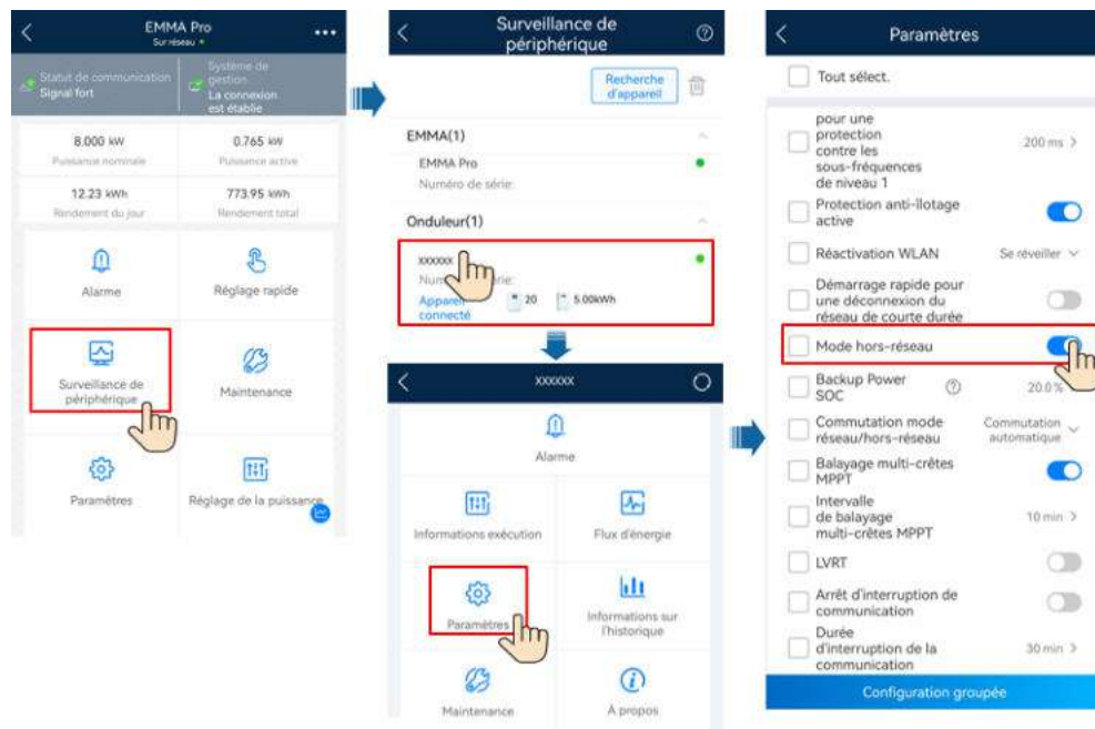
Figure 6-5 Réglage du mode hors-réseau
