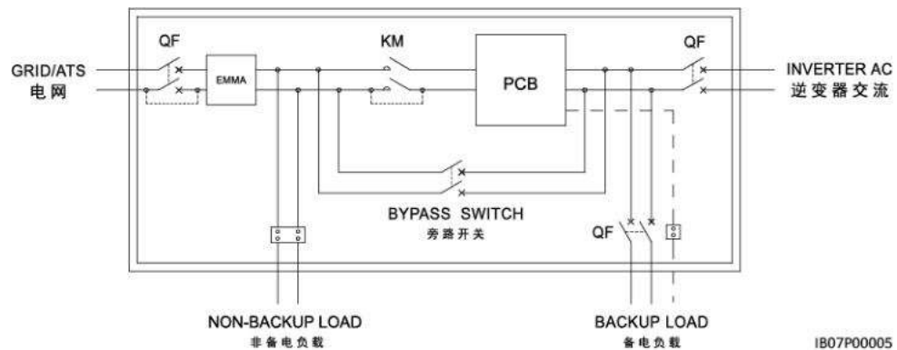
Figure 2-9 Schéma électrique du SmartGuard
