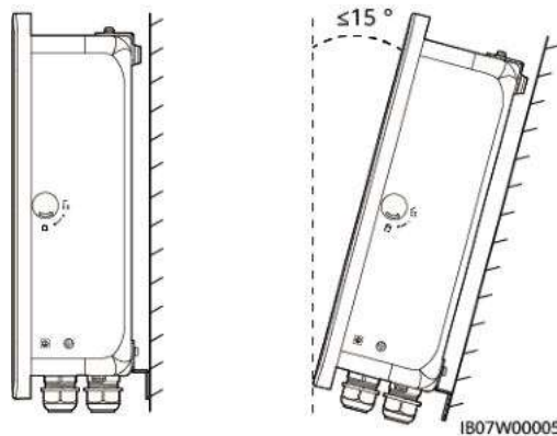
Figure 4-3 Angle d'installation
