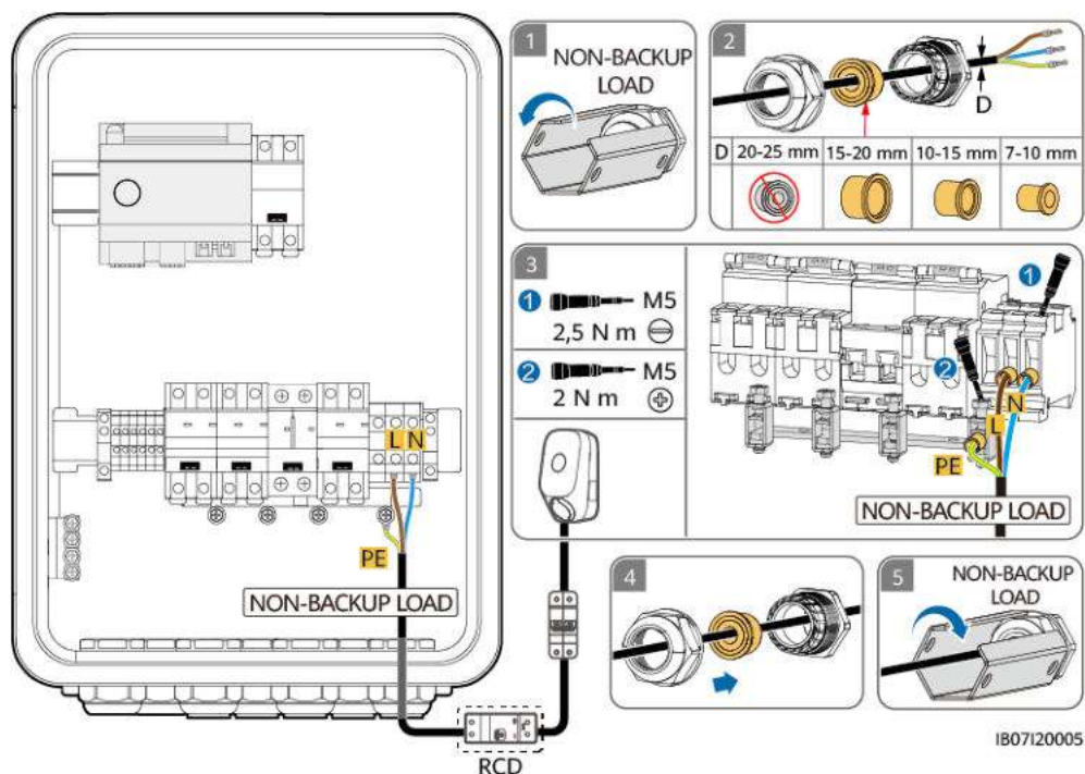
Figure 5-14 Connexion du câble d'alimentation de sortie de charge non secours (le composant dans la boîte en pointillés est optionnel)
