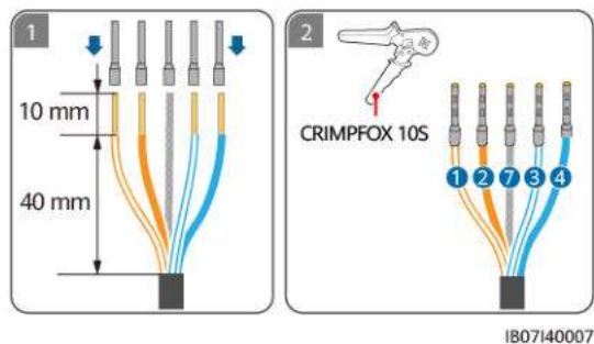
Figure 5-21 Sertissage des bornes d'extrémité du cordon pour le câble de signal
