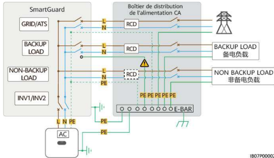
Figure 2-3 Schéma de câblage résidentiel du SmartGuard-63A-S0 (les lignes pointillées indiquent les connexions de câble optionnelles)
