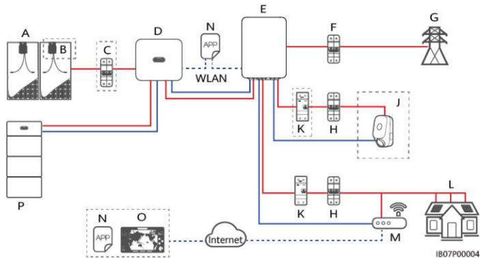
Figure 2-5 Mise en réseau (composants optionnels indiqués par des cadres en pointillés)
