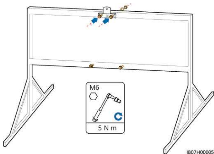
Figure 4-9 Fixation du soutien de montage
