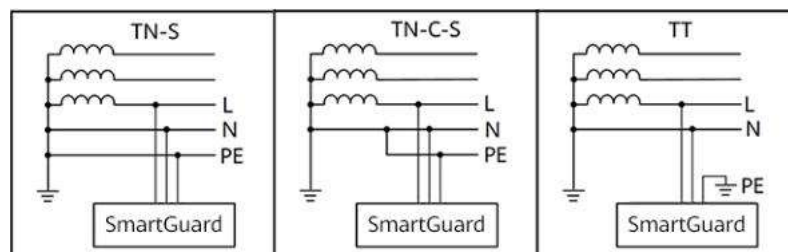
Figure 2-6 Systèmes de mise à la terre
