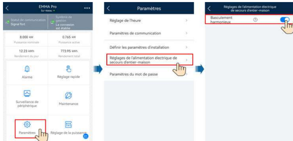
Figure 6-4 Paramétrage du basculement harmonieux
