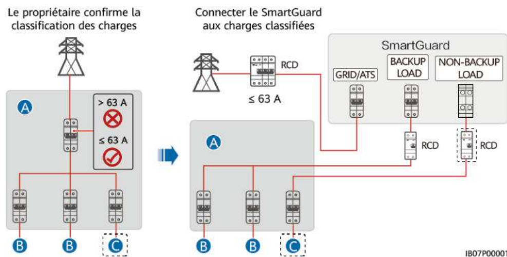
Figure 2-2 Classification des charges résidentielles (composants optionnels indiqués par des cadres en pointillés)
