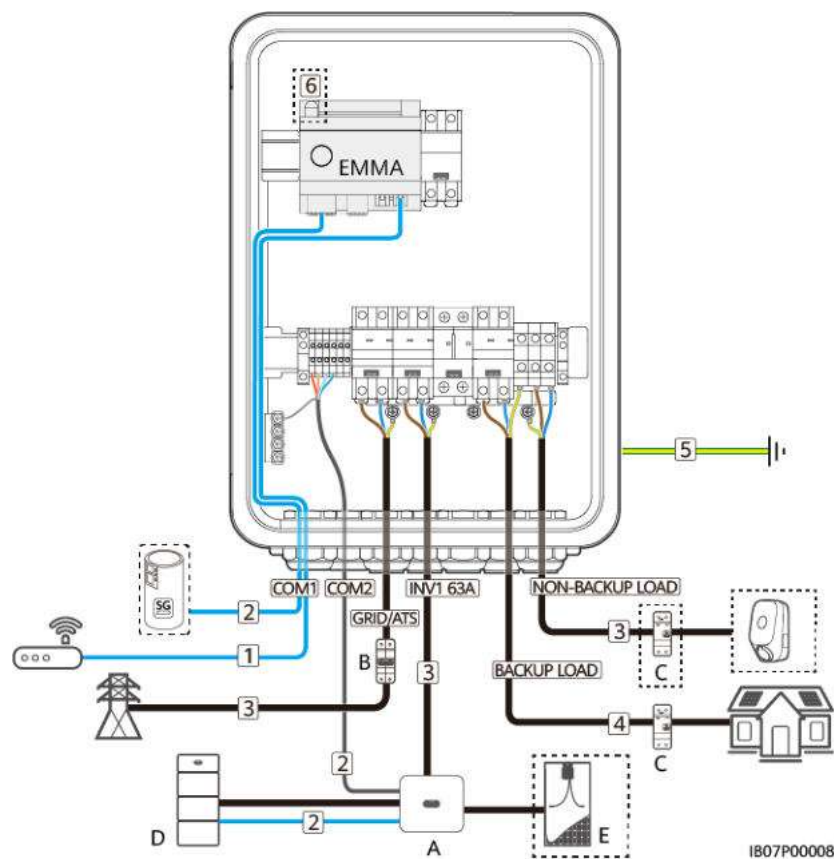
Figure 5-1 Connexions des câbles (configuration optionnelle indiquée par des cadres en pointillés)
