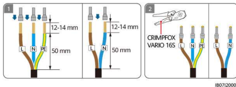
Figure 5-6 Sertissage des bornes d'extrémité du cordon CA
