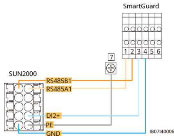
Figure 5-20 Connexion des câbles aux port COM sur le SmartGuard
