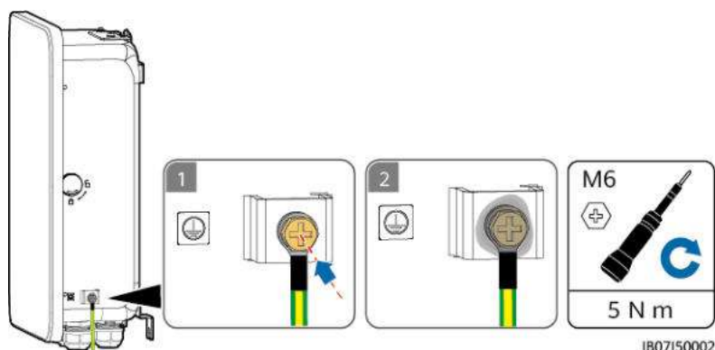
Figure 5-3 Connexion du câble PE
