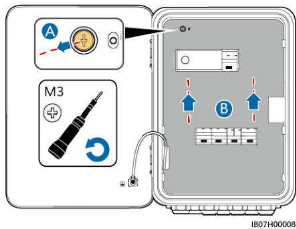
Figure 5-5 Ouverture du couvercle du compartiment de maintenance
