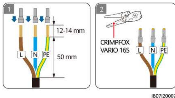
Figure 5-10 Sertissage des bornes d'extrémité du cordon CA SmartGuard-63A-S0
