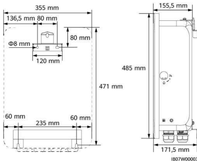
Figure 4-1 Dimensions du support de montage
