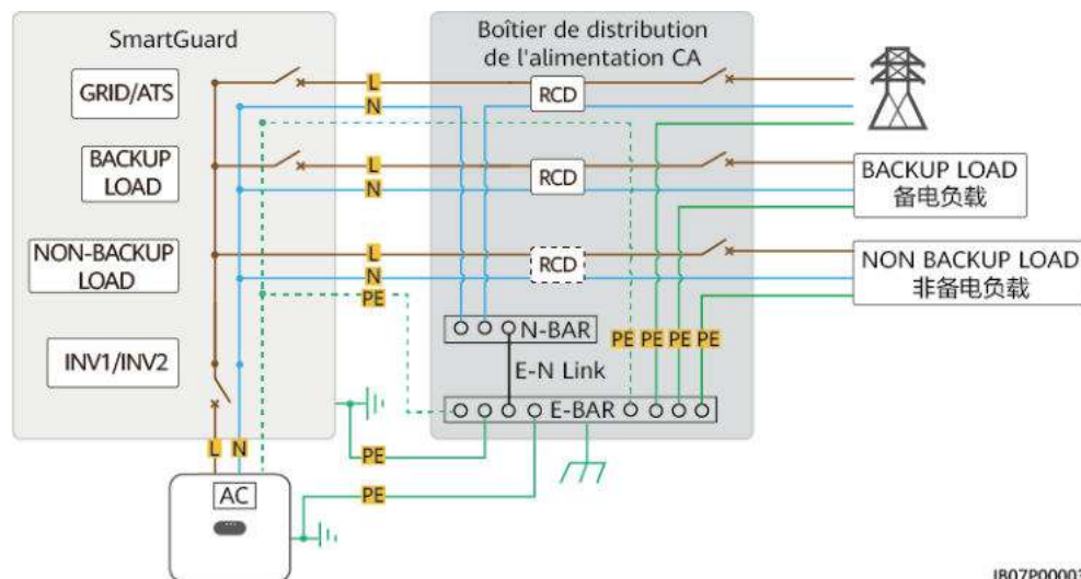
Figure 2-4 Schéma de câblage résidentiel du SmartGuard-63A-AUS0 (les lignes pointillées indiquent les connexions de câble optionnelles)
