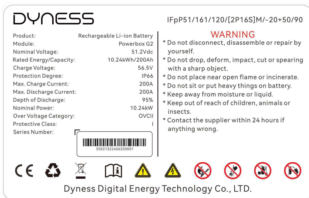
Figure 1 - 1 Plaque signalétique du système de stockage d'énergie par batterie
