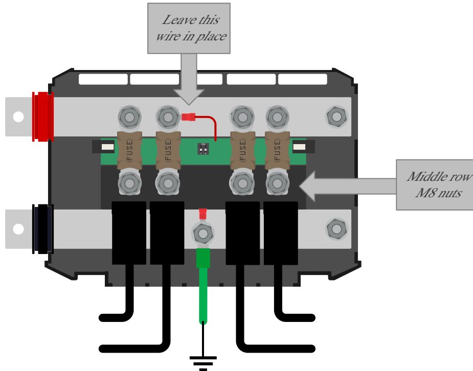
Mise en place des fusibles du distributeur Lynx
