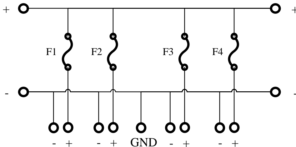
Schéma de branchement du distributeur Lynx
