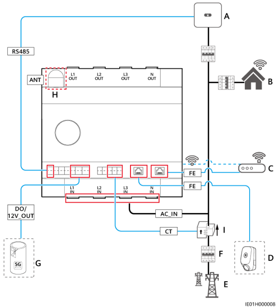
Figure 5-2 Diagramme de connexion des câbles : connexion CT externe (courant > 63 A)
