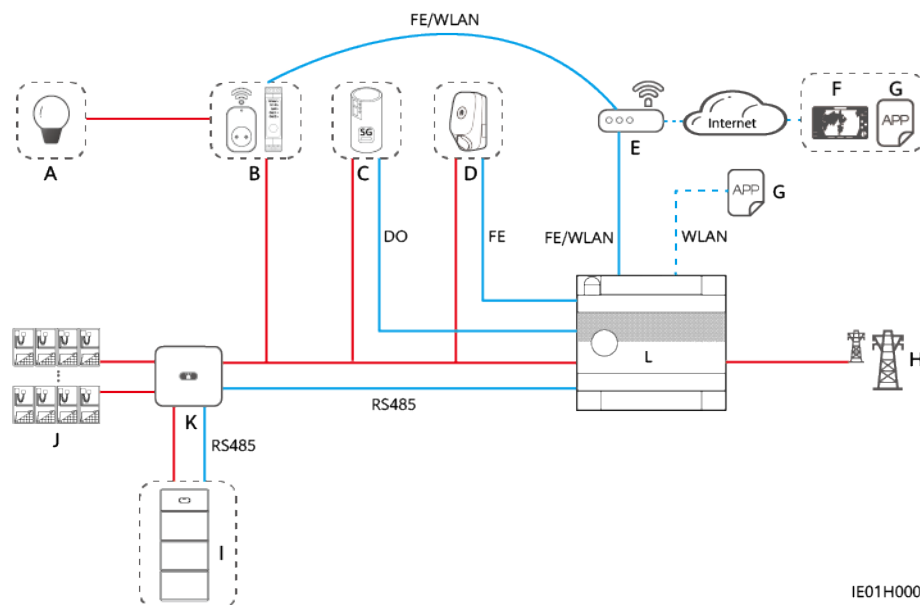
Figure 2-2 Diagramme de mise en réseau (en utilisant l'EMMA-A02 comme exemple)
