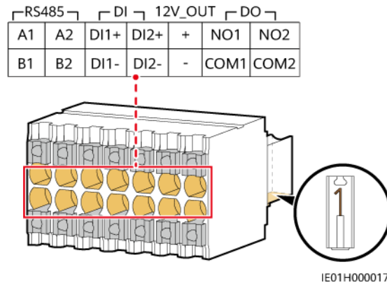
Figure 5-9 Connecteur 14 broches
