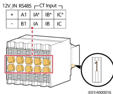
Figure 5-5 Connecteur 10 broches
