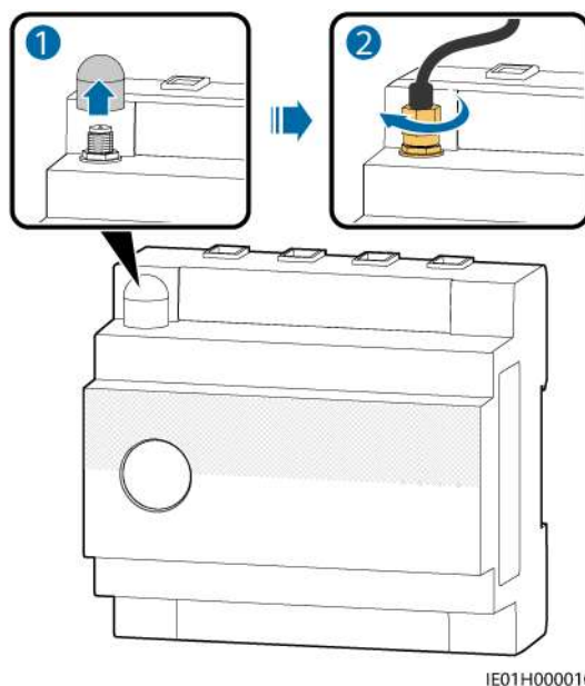
Figure 5-15 Installation d'une antenne WLAN
